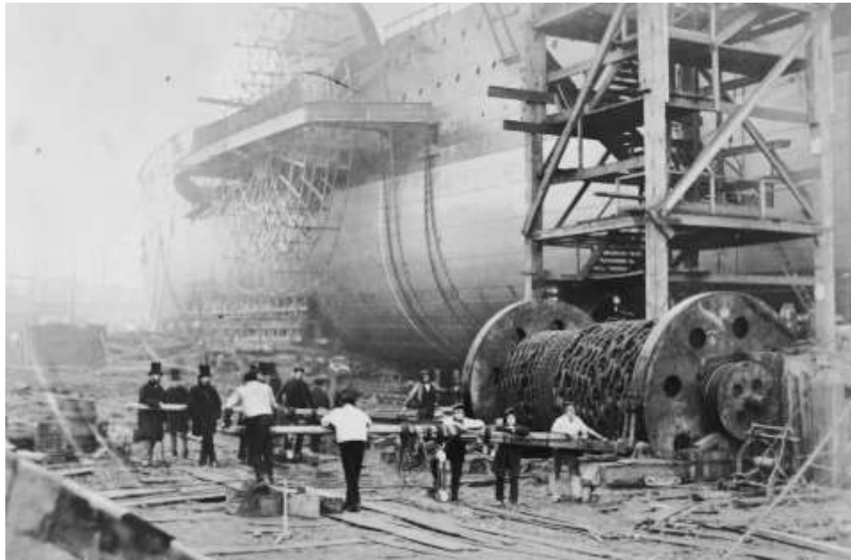
Строительство парохода Great Eastern
